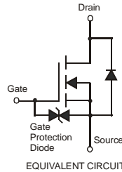
SOT-523
